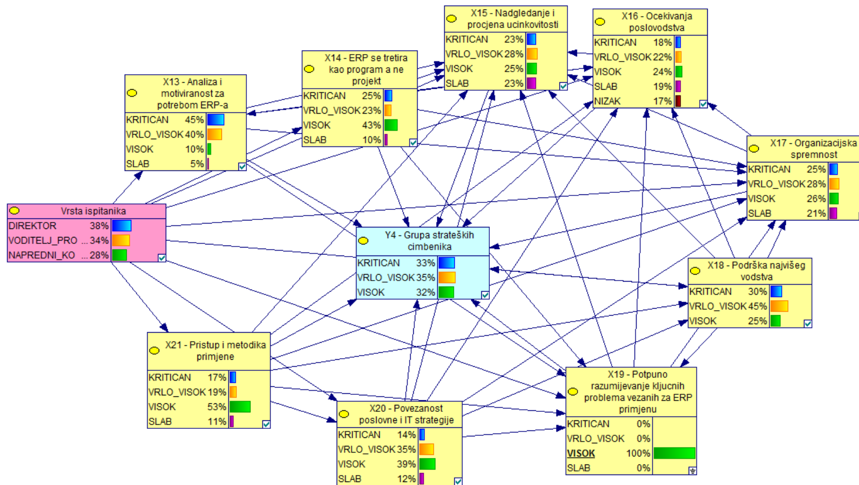
Slika 69: Bayesova mreža utjecaja ekstremnih vrijednosti po stanjima varijable „potpuno razumijevanje ključnih problema vezanih za ERP primjenu“ (X19), visok=100%, na vrijednosti stanja varijabli kritičnih čimbenika (X13, X14, X15, X16, X17, X18, X20, X21) i grupu kritičnih čimbenika Y4
