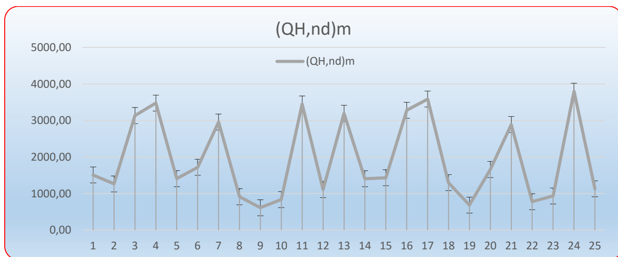
Slika 7-6. Potrošnja energije stvarnog stanja (kWh) – strop iznad grijanog prostora
