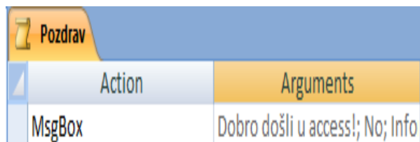
Slika 29: MsgBox
