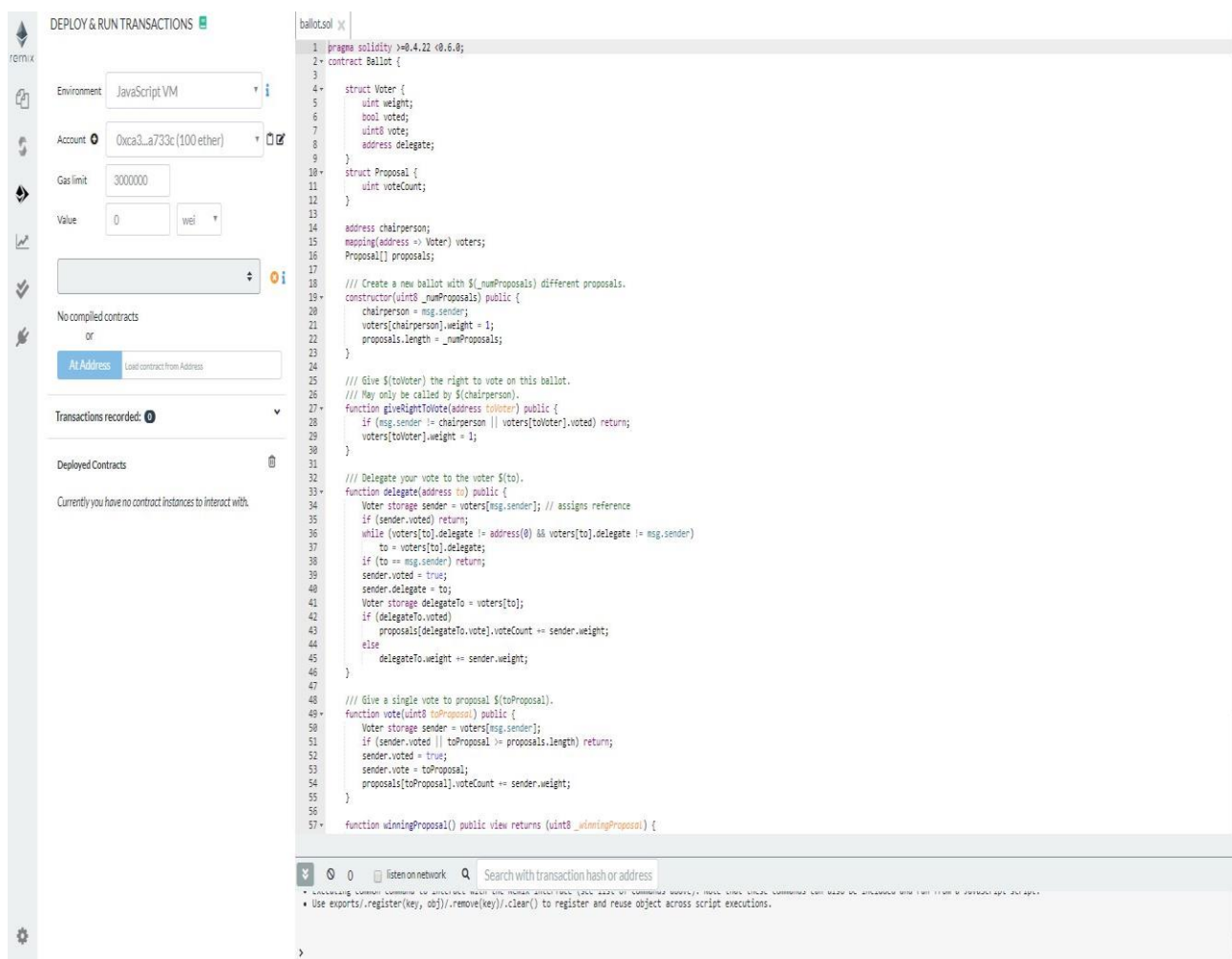
Slika 19. Primjer ugovora napisanog u Remix IDE ( http://remix.ethereum.org/ )
