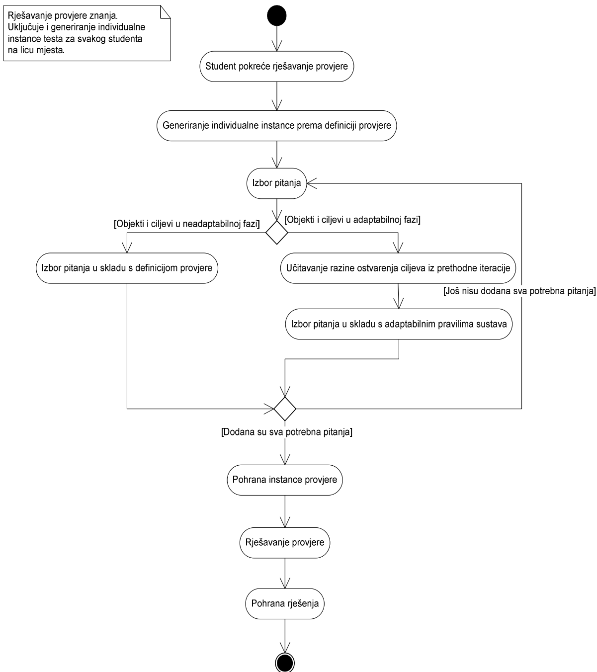
Slika 22. Koraci generiranja i rješavanja pojedinačnih instanci testova
