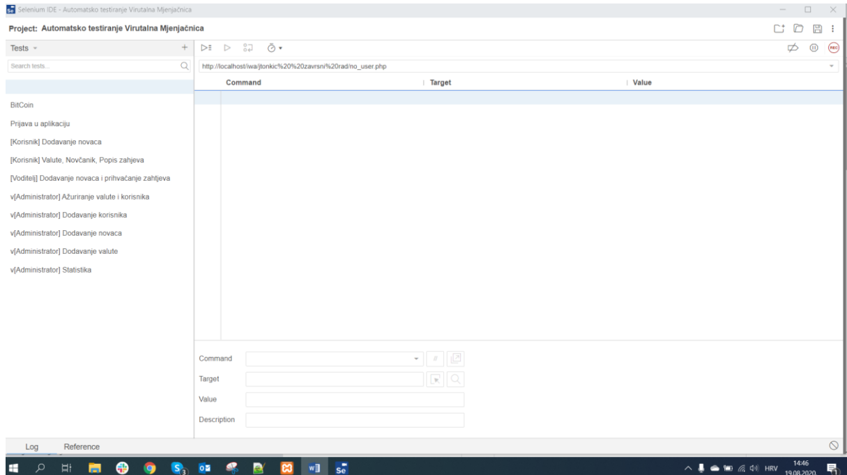
Slika 17. Selenium IDE
