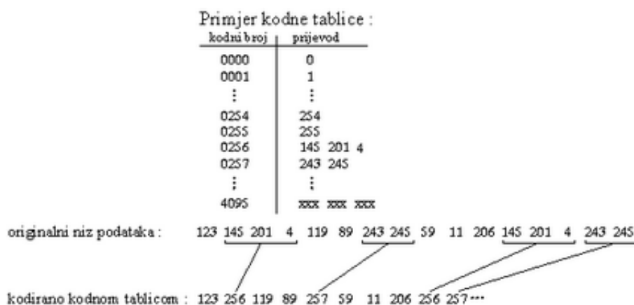
Slika 20. Entropijsko kodiranje (Mihić, Štuka, Vuksanović, 2014., str. 10)
