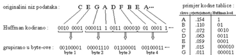
Slika 19. Primjer Huffman kodiranja (Mihić, Štuka, Vuksanović, 2014., str. 9)
