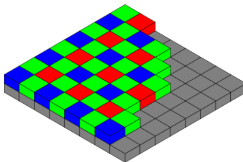
Slika 3. Bayer filter (Strgar Kurečić, 2017.)
