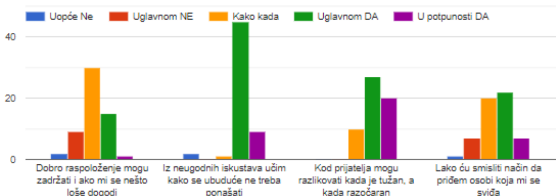
Slika 6: Tvrdnje 1-4
