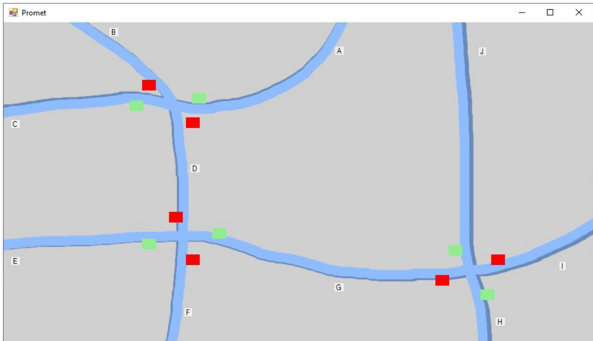
Slika 5: Forma s raskrižjima u početku simulacije (isječak zaslona)
