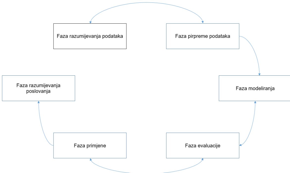
Slika 43: Metodologija implementacije modela stabla odlučivanja za PT BPR X (Izvor: vlastita izrada prema [61, str. 4])
