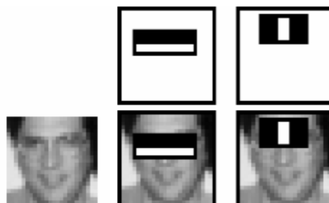
Slika 32: Primjer značajki (Izvor: OpenCV)
