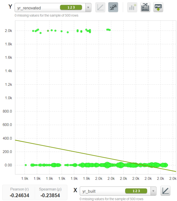
Slika 6: Korelacija varijabli yr_built i yr_renovated (Izvor: vlastita izrada)
