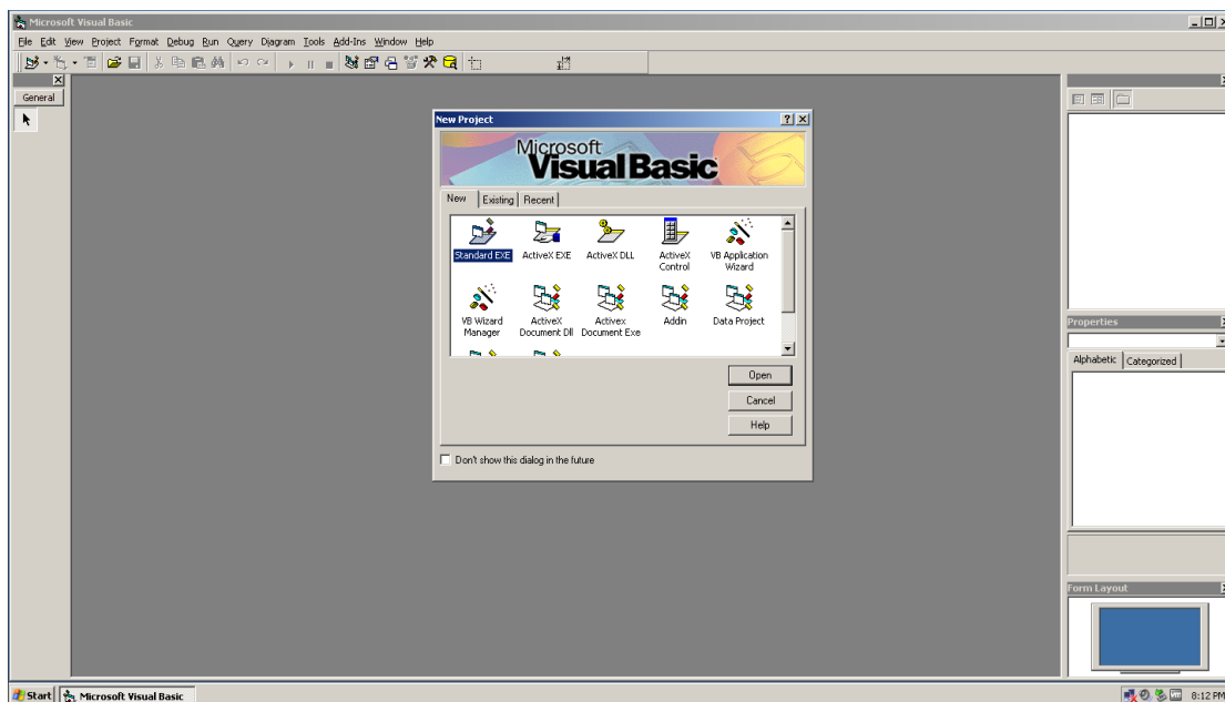
Slika 2: Visual Basic 6 [4]
