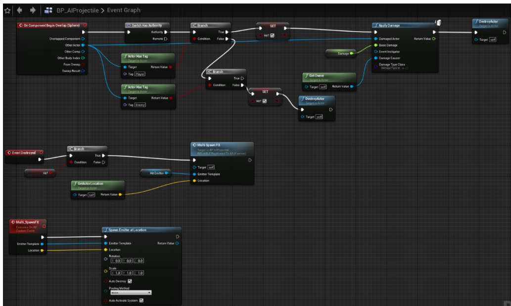
Slika 78: „BP_AIProjectile“
