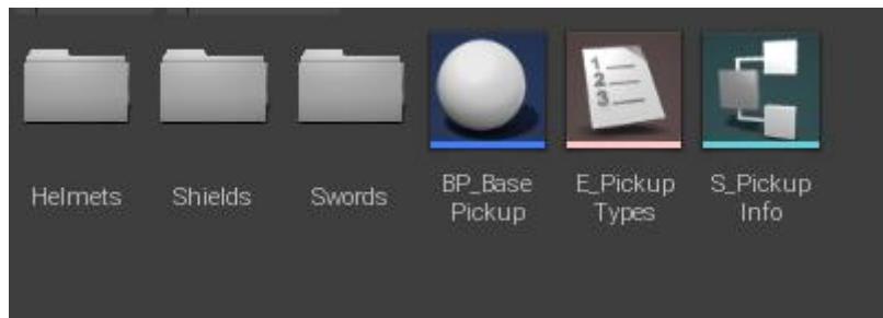
Slika 5: Mapa „Pickups“
