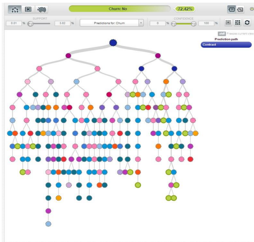
Slika 9: Stablo odlučivanja
