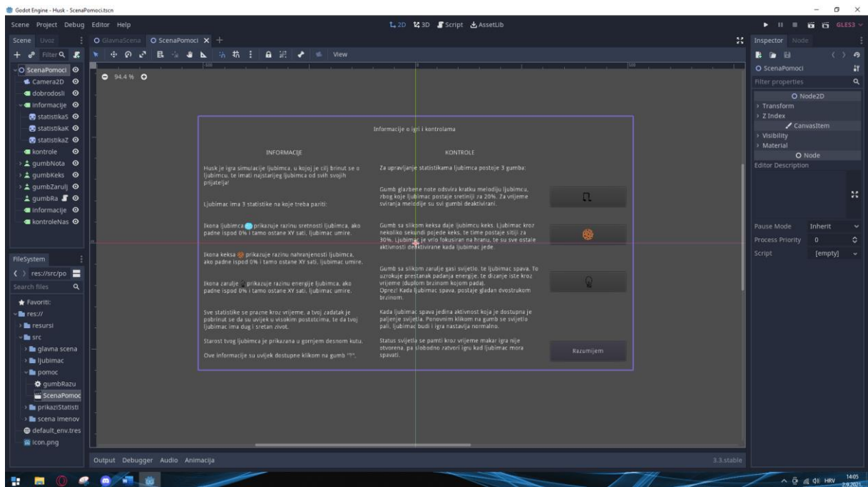
Slika 35: Scena pomoći
