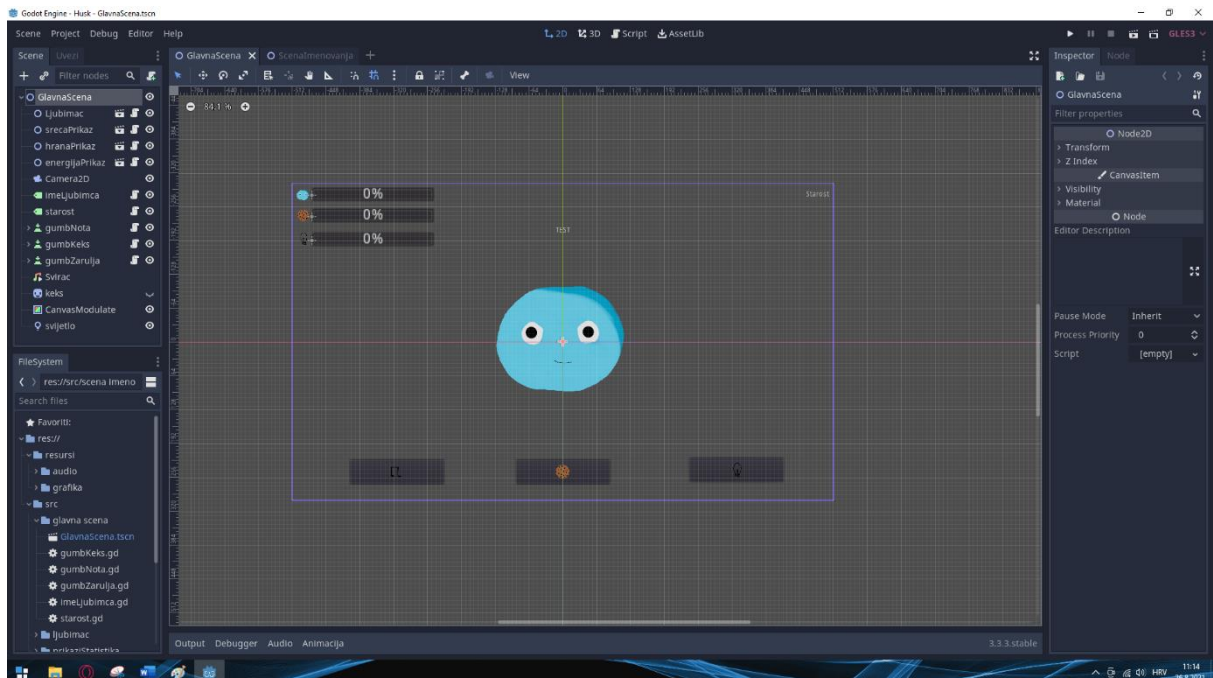
Slika 33: Glavna scena
