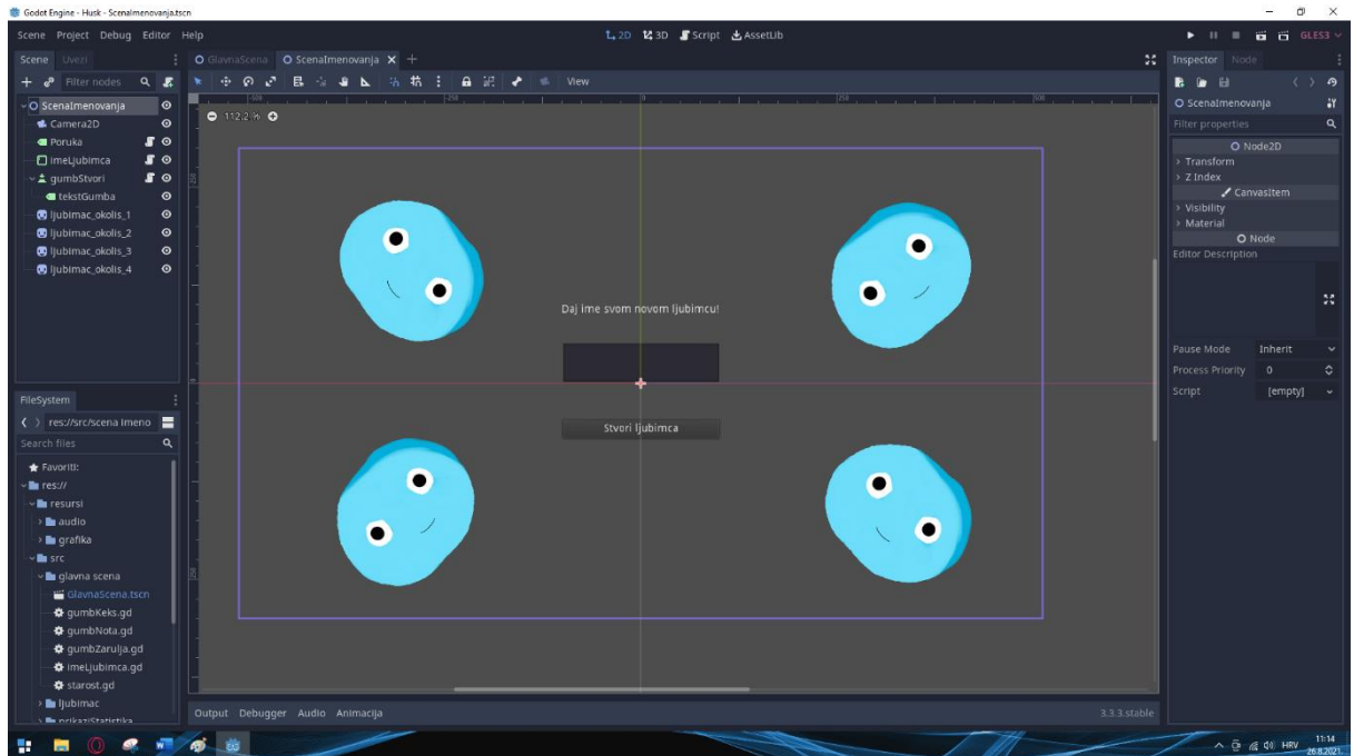
Slika 34: Scena Imenovanja
