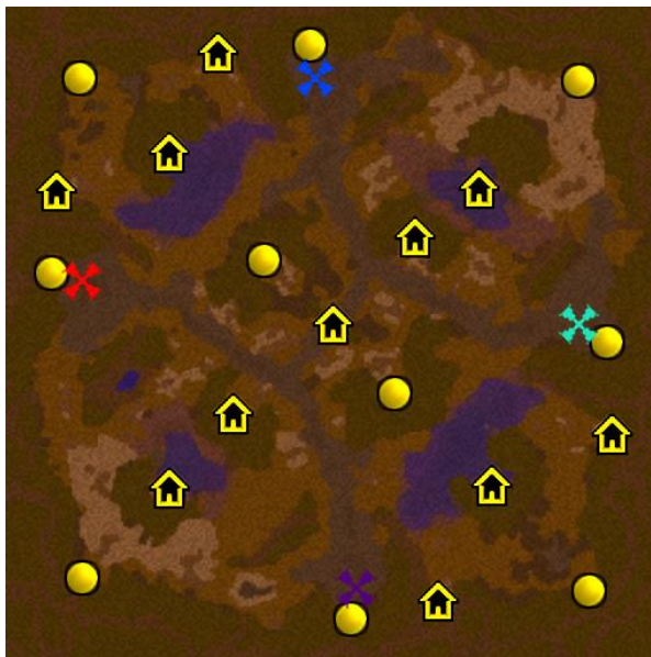
Slika 11. Simetrična mapa [20]
