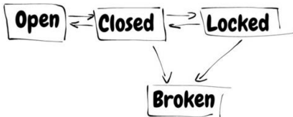
Slika 10. Stanja vrata [18]
