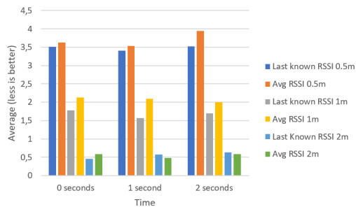
(a) Vrijednosti varijable Average
