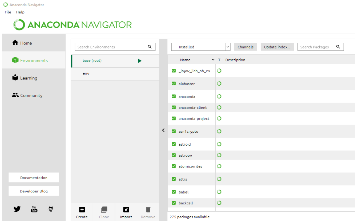
Slika 6: Anaconda Navigator
