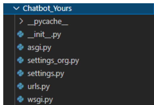
Slika 7: Chatbot_Yours
