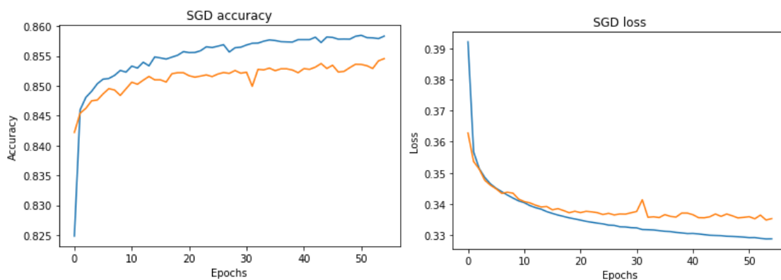
Slika 85 Točnost i vrijednost funkcije gubitka po epochama SGD
