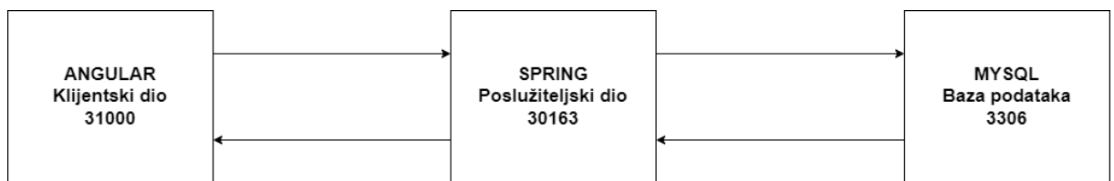
Slika 17. Arhitektura aplikacije za vođenje autoškole [Autorski rad]
