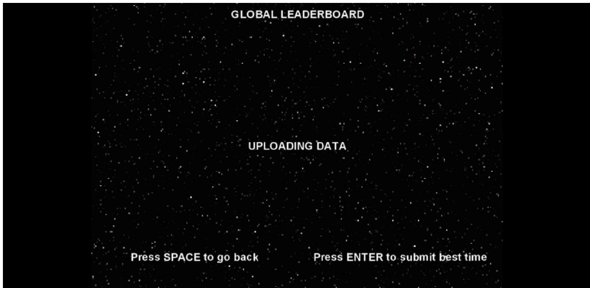
Slika 7. Slanje rezultata
