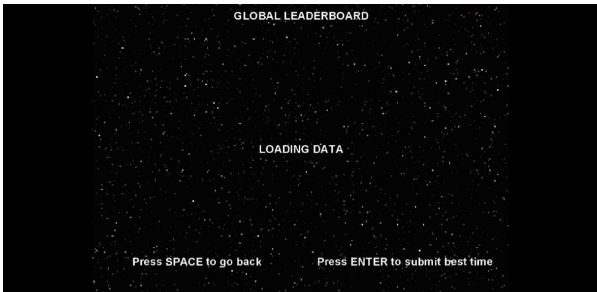
Slika 8. Dohvaćanje rezultata
