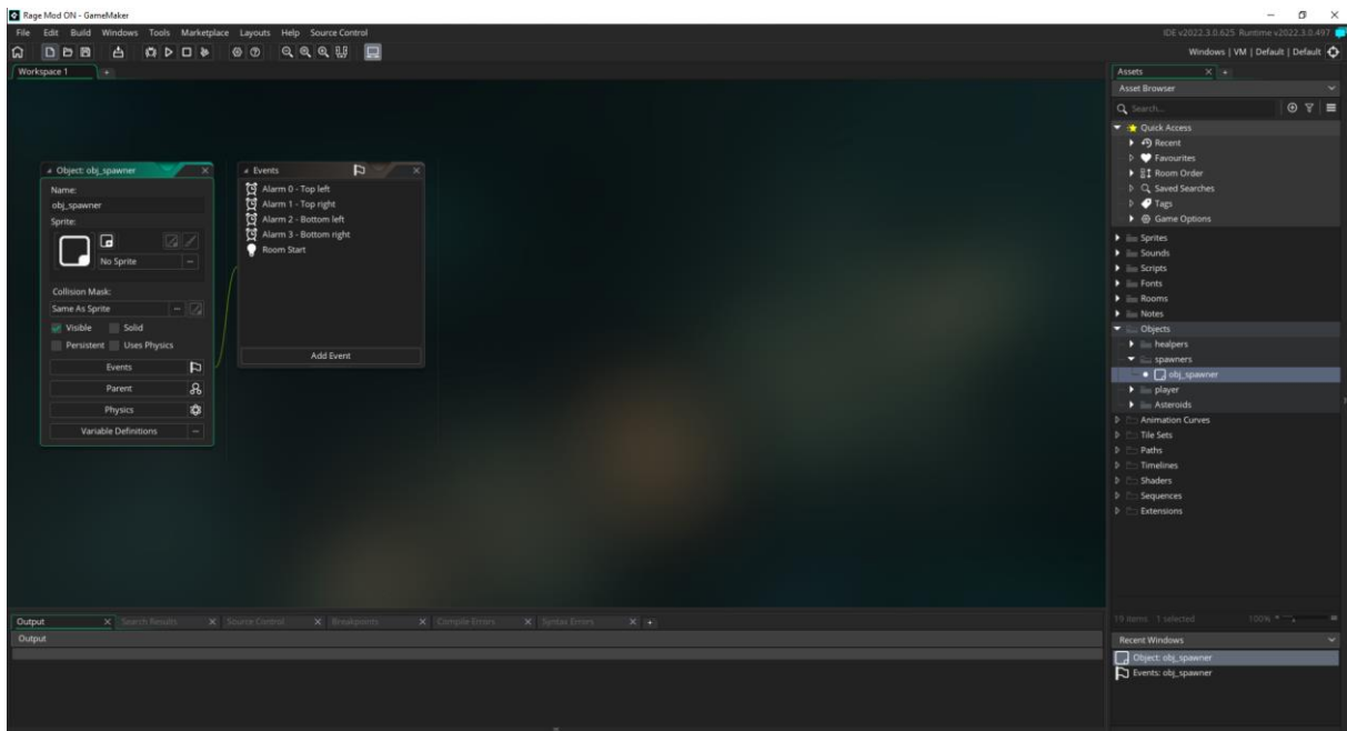
Slika 1. Sučelje GameMaker-a
