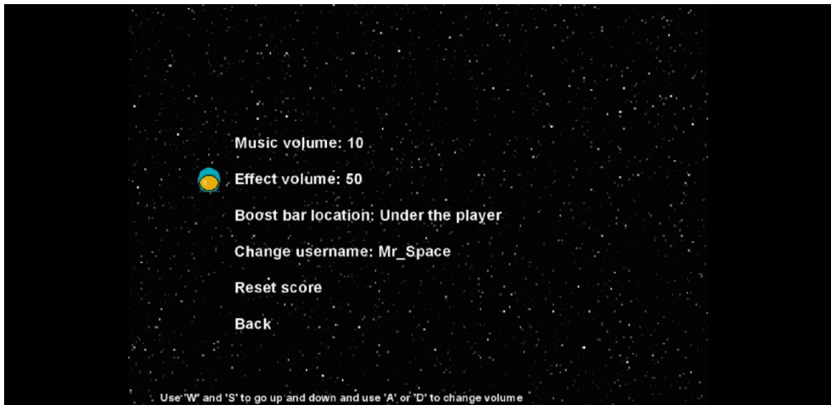
Slika 12. Izbornik opcija
