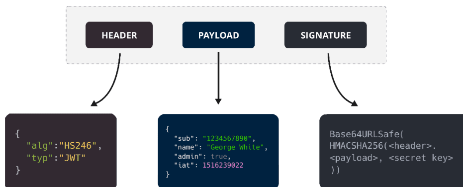
Slika 45. Struktura JWT-a [104]
