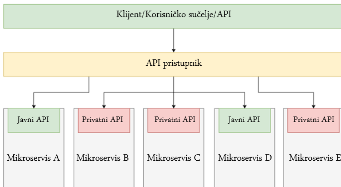
Slika 9. API pristupnik [28].
