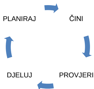
Slika 2.: Shewhartov ciklus (Izvor: Šiško Kuliš, Mrduljaš, 2009)
