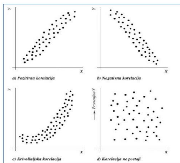
Slika 5.: Dijagram rasipanja za vrste korelacije između pojava (Izvor: Čelar i dr., 2014)
