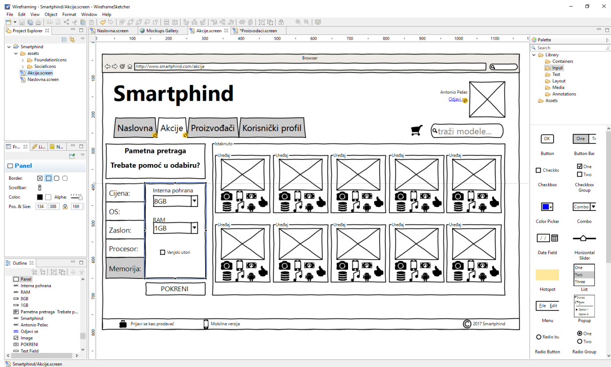
Slika 34. Ekran „Akcije“ u alatu WireframeSketcher
