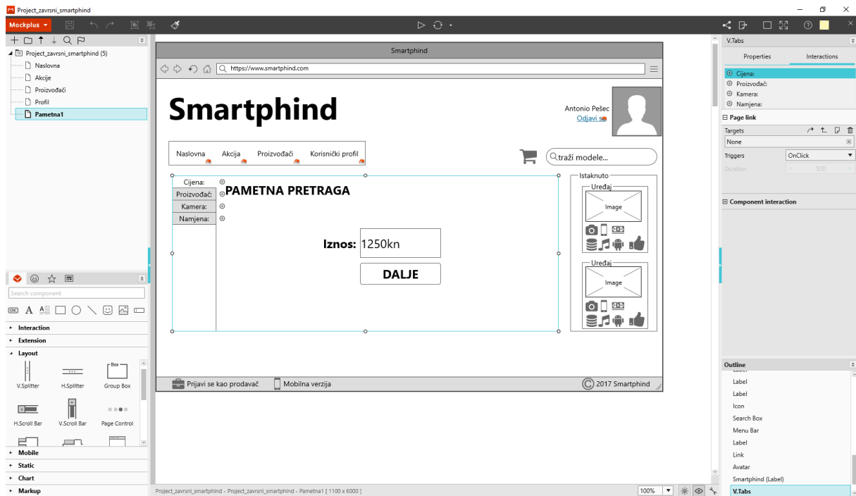
Slika 20. Ekran „Pametna1“ u alatu Mockplus
