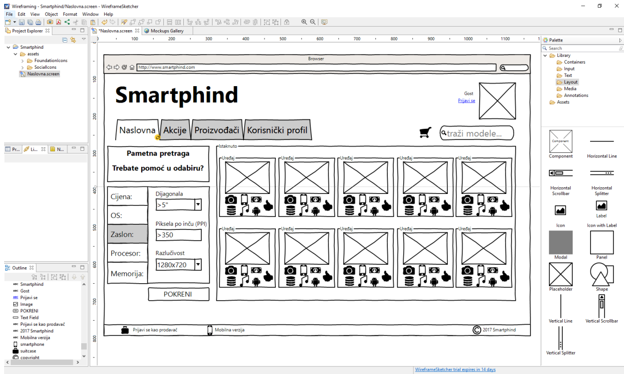
Slika 33. Ekran „Naslovna“ u alatu WireframeSketcher
