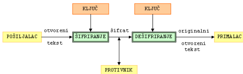
Slika 3: Proces enkripcije i dekripcije ključevima [11]
