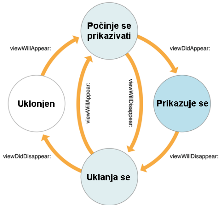
Slika 6 Životni ciklus ViewController-a (Prema:
