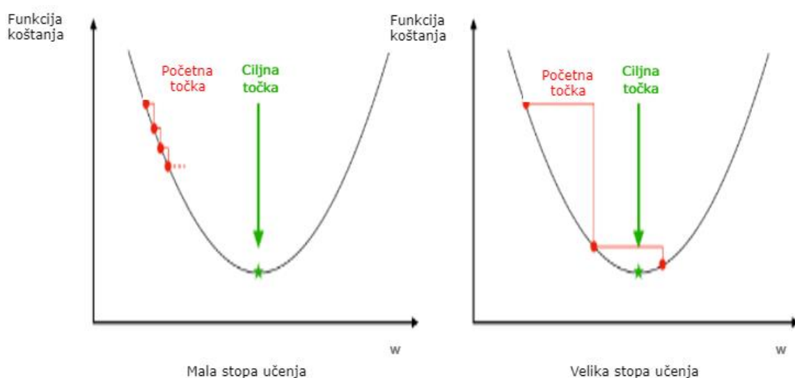
Slika 8: Usporedba stopi učenja za gradijenti spust
