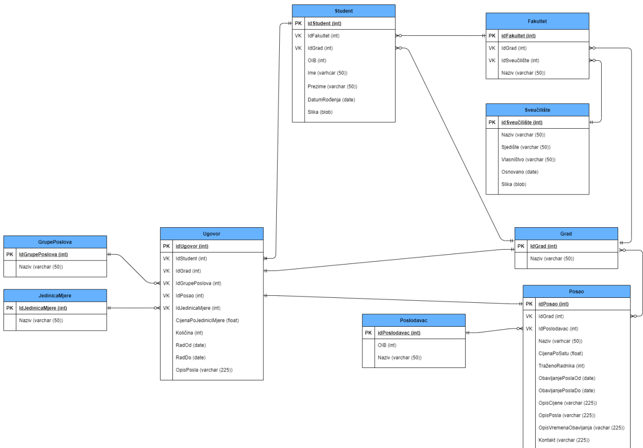
Slika 19. ERA model (Samostalna izrada)
