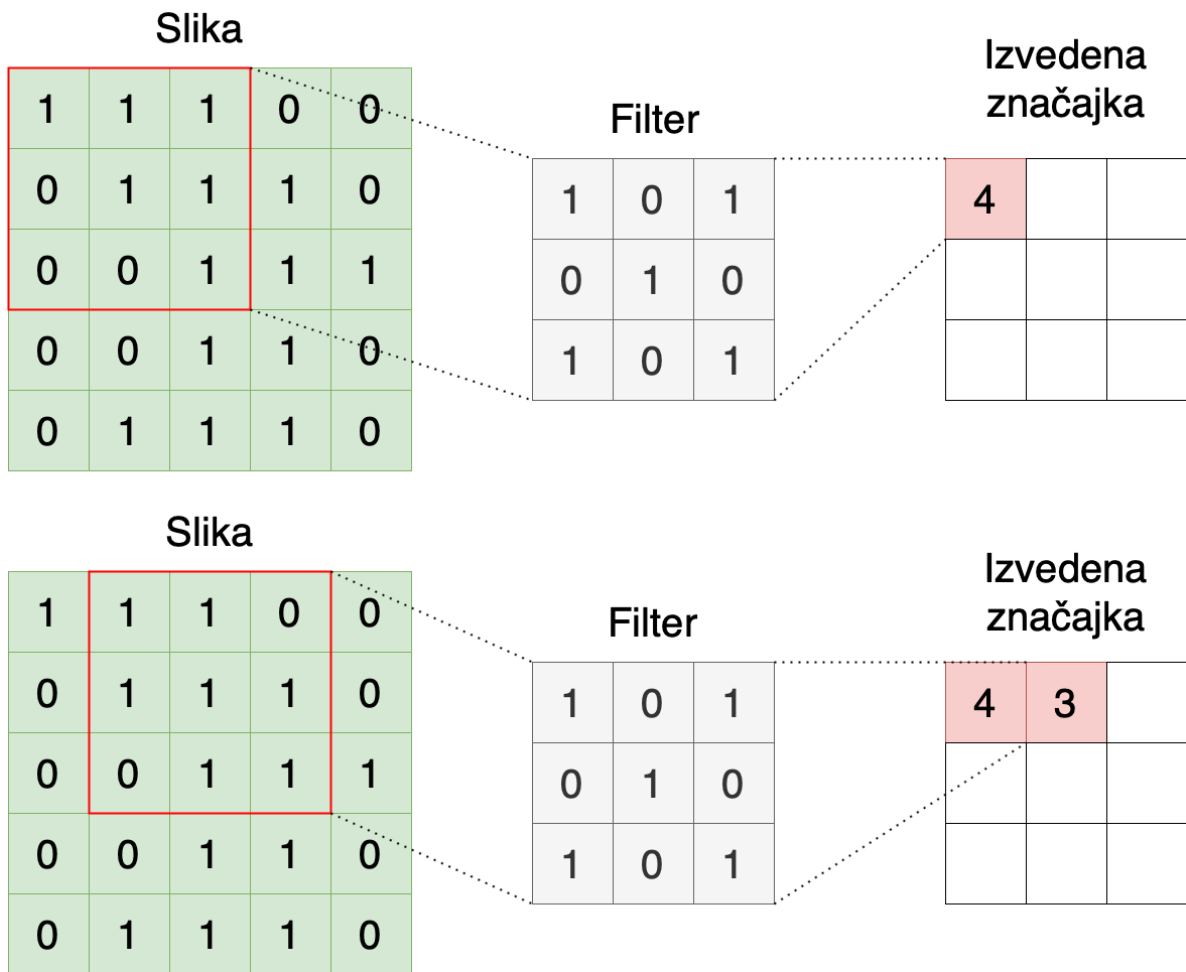
Slika 21. Izvršavanje konvolucije uz pomoć filtera (Patterson & Gibson, 2019)
