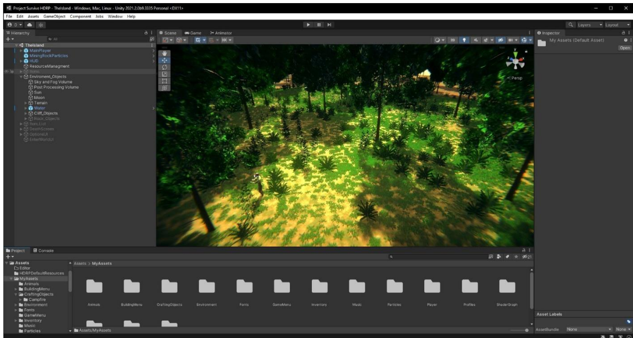
Slika 1. Unity sučelje
