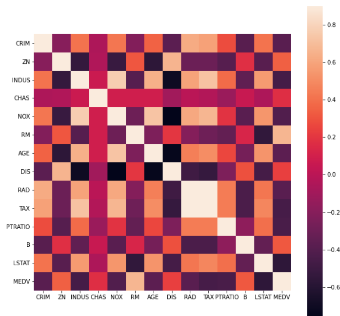
Slika 127 Korelacijska matrica
