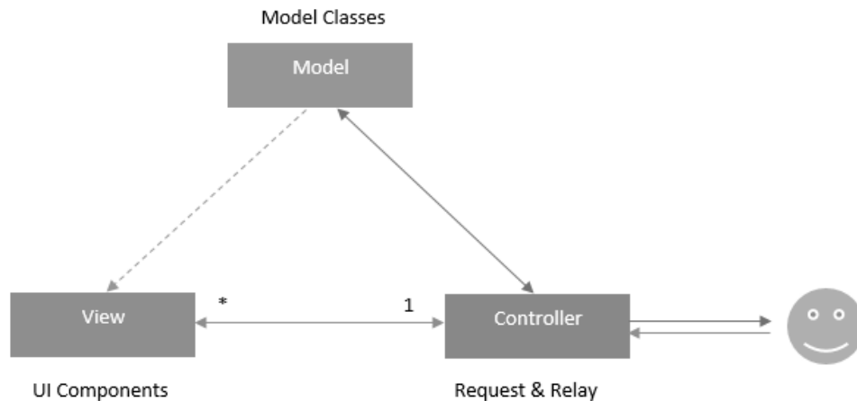
Slika 3: MVC arhitektura, [13]
