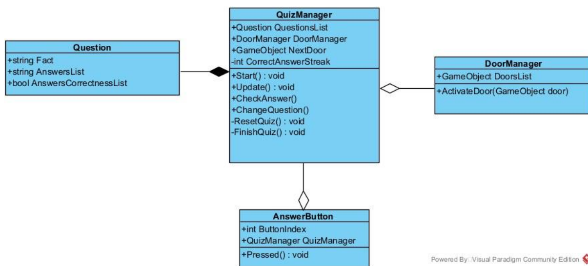
Slika 15. Dijagram klasa
