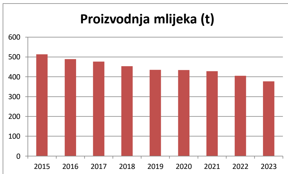
Grafikon 2 Prikaz proizvedenog mlijeka u Hrvatskoj
