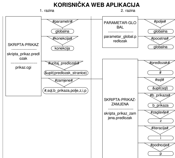
Slika 5.10: Dijagram metaskriptata generatora korisničkih web aplikacija
