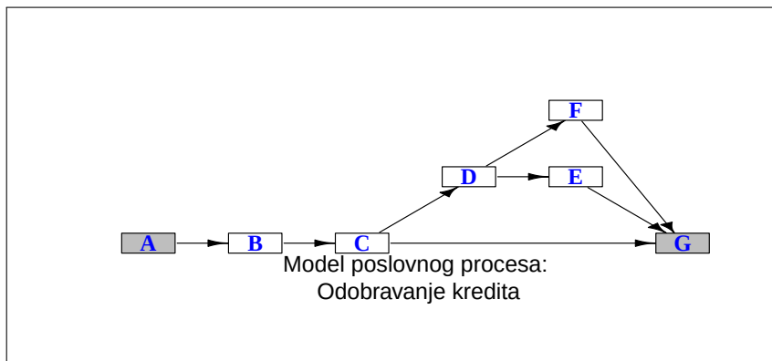
Slika 6.2: Odobravanje kredita : matematički graf poslovnog procesa
