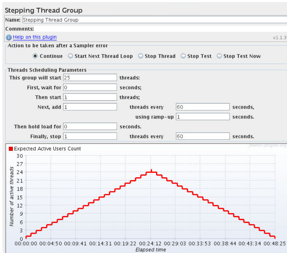
Slika 7.39. - Prikaz parametara u alatu Apache JMeter za prvi eksperiment
