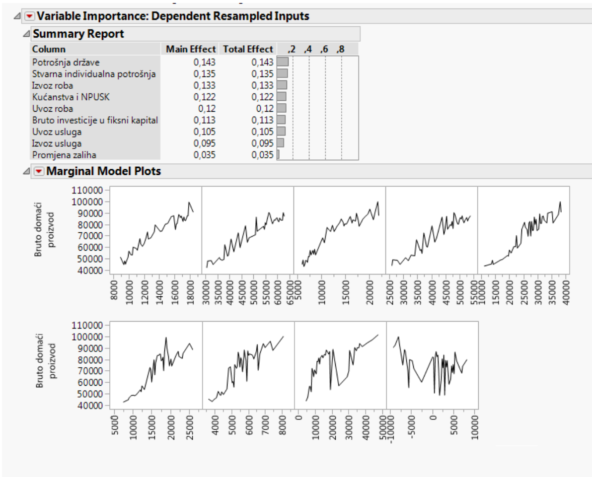
Slika 25: Prikaz važnosti varijabli (Izvor: autorski rad)
