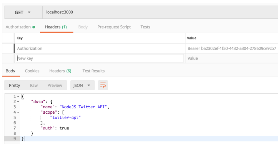
Slika 7 - Odgovor metode za provjeru statusa ključa
