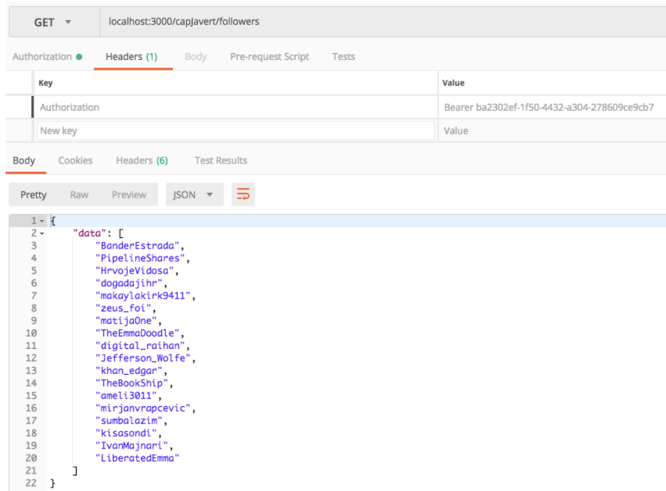
Slika 9 - Odgovor metode za ispis pratitelja korisnika
