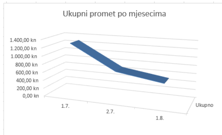
Slika 20:Linijski grafikon
