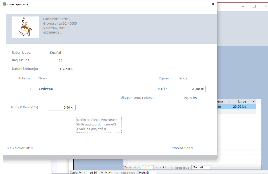
Slika 10: Izvještaj računa
