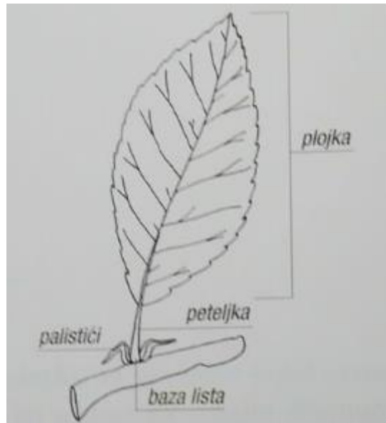
Slika 1 Građa lista, [19]
