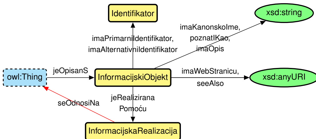
Slika 66: Uzorak informacijskog objekta (prema Krishnathi, Hu i Arko (2015))
