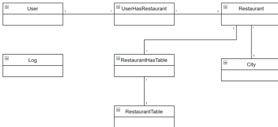
Slika 17 ERA model baze podataka
