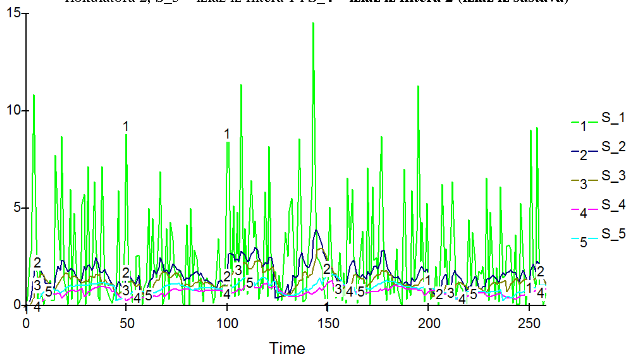
Slika 49. Izlazne simulirane vrijednosti koncentracije organske tvari iz dijelova sustava za pročišćavanje otpadne vode u vodu za ljudsku potrošnju bez izlaza iz bioeracijskog spremnika 1 (S_1 – izlaz iz bioeracijskog spremnika 2, S_2 – izlaz iz flokulatora 1, S_3 – izlaz iz flokulatora 2, S_5 – izlaz iz filtera 1 i S_4 – izlaz iz filtera 2 (izlaz iz sustava) )
