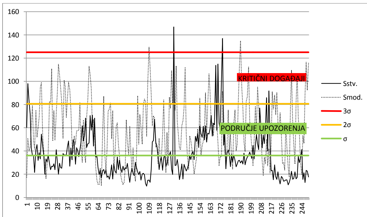
Slika 35. Kontrolna karta za organsku tvar na mjernom mjestu 1
