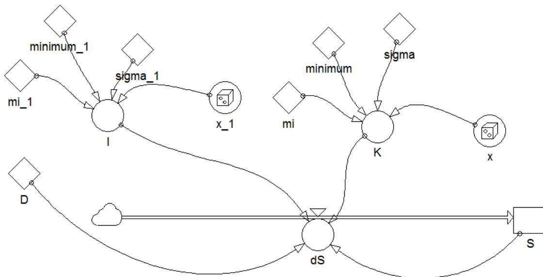
Slika 16. Računalni model pročišćavanja vode od organske tvari u bioeracijskom spremniku
