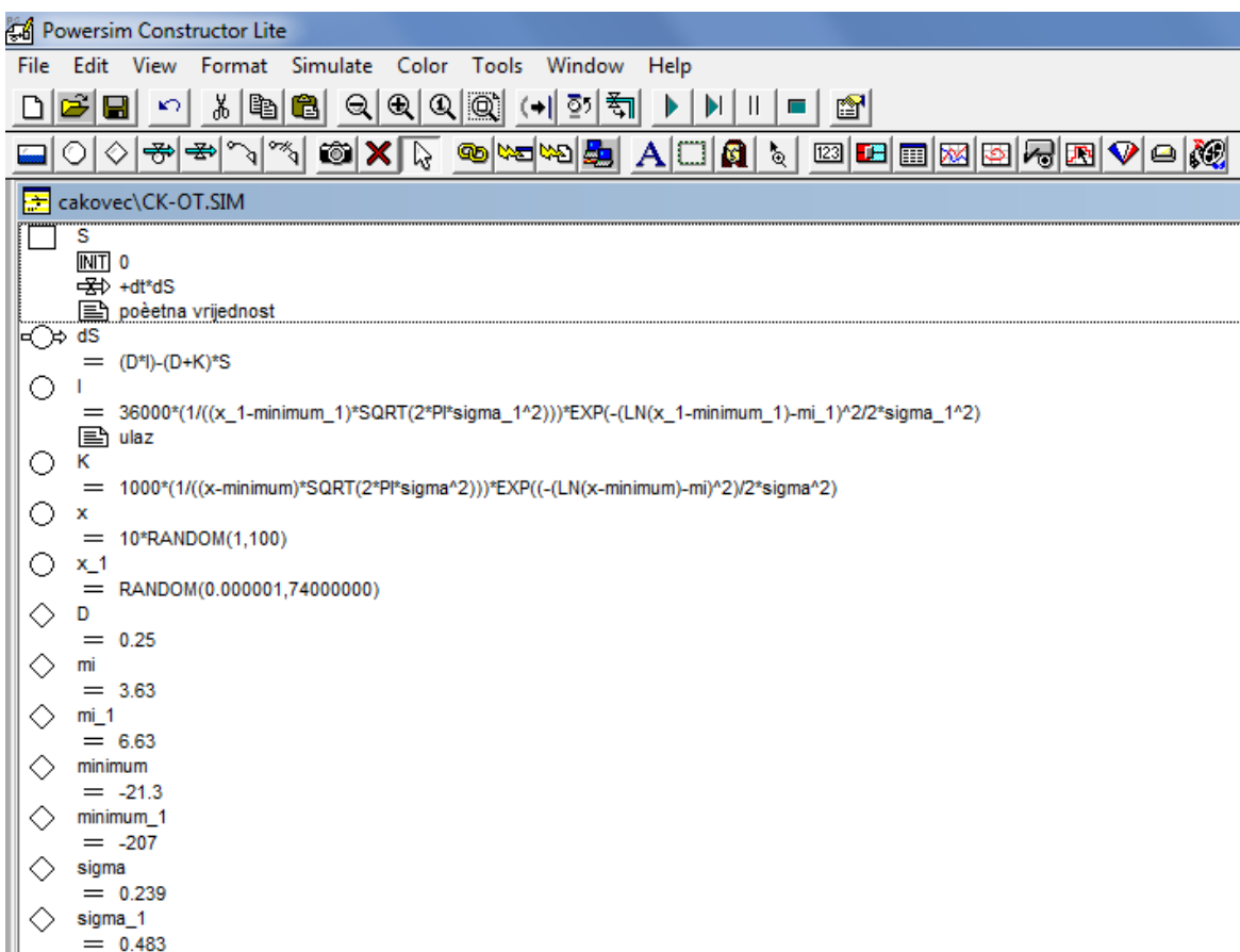
Slika 17. Jednadžbe modela pročišćavanja vode od organske tvari u bioeracijskom spremniku
