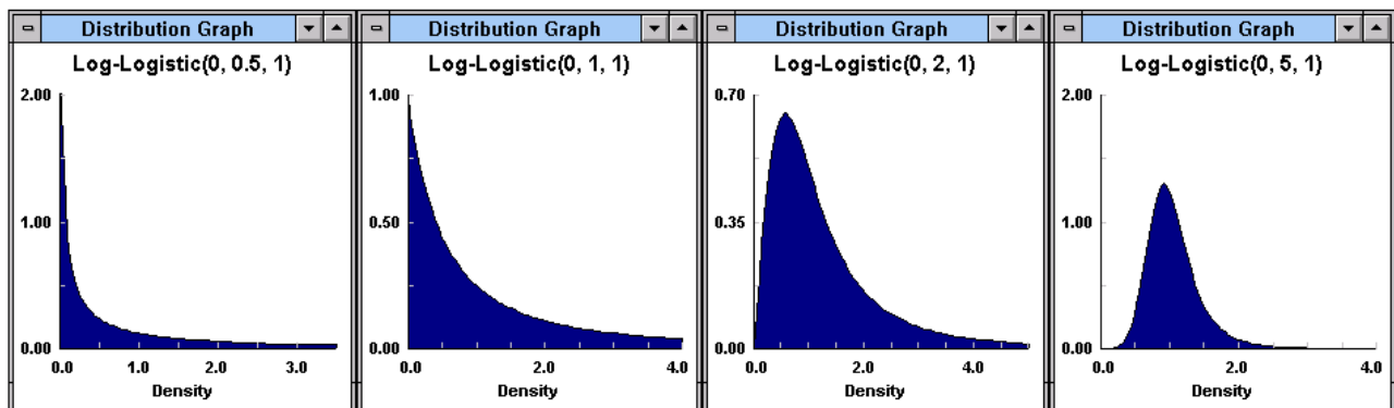
Slika 6. Promjena oblika Log – logistične distribucije prema promjeni parametra oblika (preuzeto: Stat Fit )
