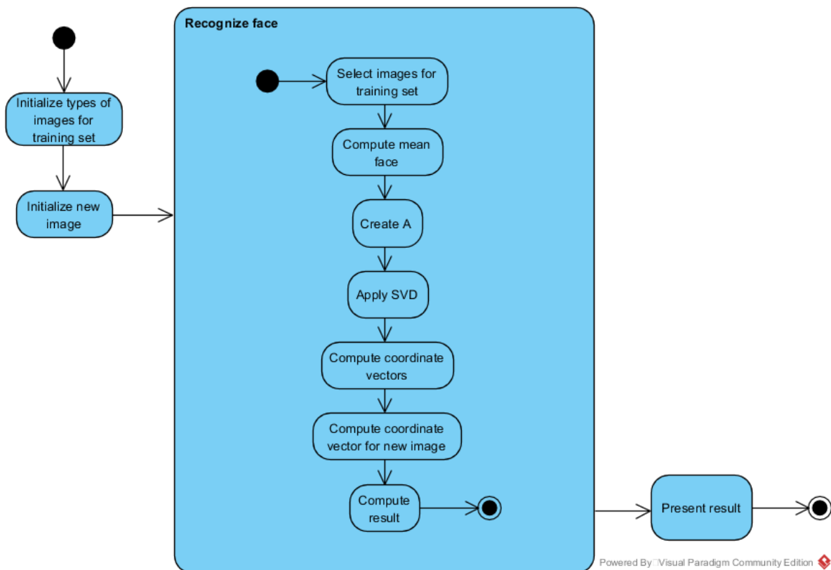
Slika 13: Dijagram aktivnosti za postupak prepoznavanja jednog novog lica
