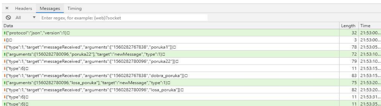
Slika 16: Primjer poruka koje se šalju preko WebSocket protokola
