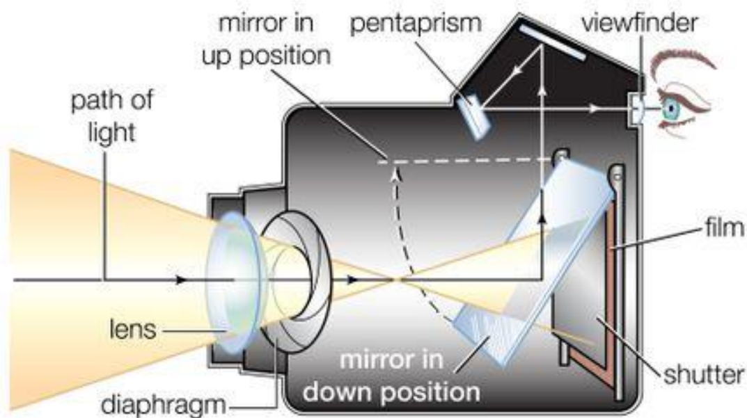
Slika 5: Princip rada DSLR fotoaparata
