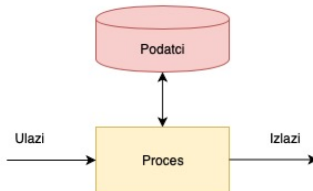
Slika 4. Transakcijski proces
